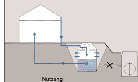
Sico-Regenspeicher, schematischer Aufbau
