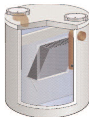
Mall-Lamellenklärer
