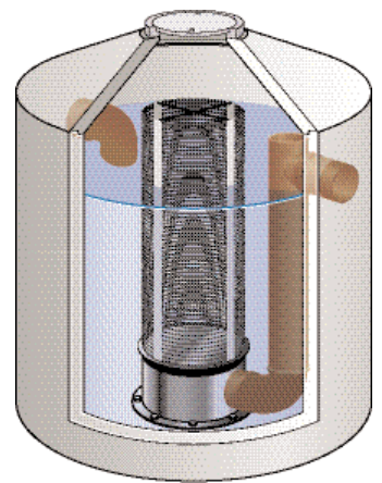
Mall-Filtertschacht
