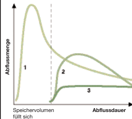
Charakteristische Abflussmengenkurven
