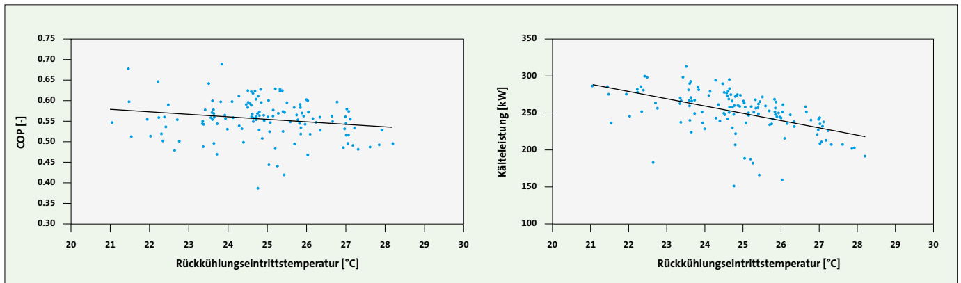
Bild 10: Messdaten zum Betrieb einer der Adsorptionskältemaschinen unter typischen Betriebsbedingungen im Sommer 2008. (Heißwassereintrittstemperaturen von 68 – 70 °C, Kaltwassereintrittstemperaturen von 13 – 14 °C und einem Heißwasservolumenstrom von 40 m 3 /h)
