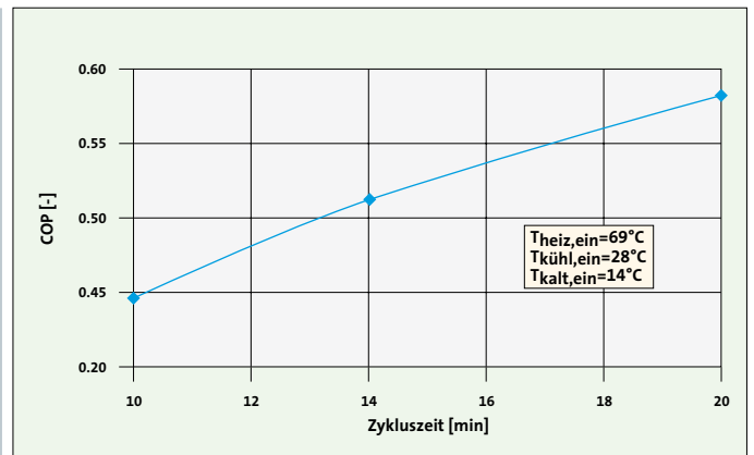
Bild 12: Simulierter thermischer COP der Adsorptionskältemaschine in Abhängigkeit von der Zykluszeit bei einem Heißwasservolumenstrom von 40 m 3 /h
